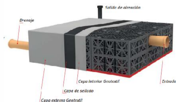
Elementos que conforman el sistema de contención o atenuación ECOBLOC GRAF
